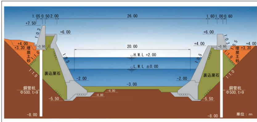
■断面図（イメージ）
