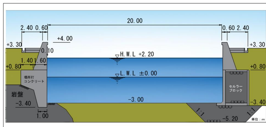
■断面図 (イメージ)
