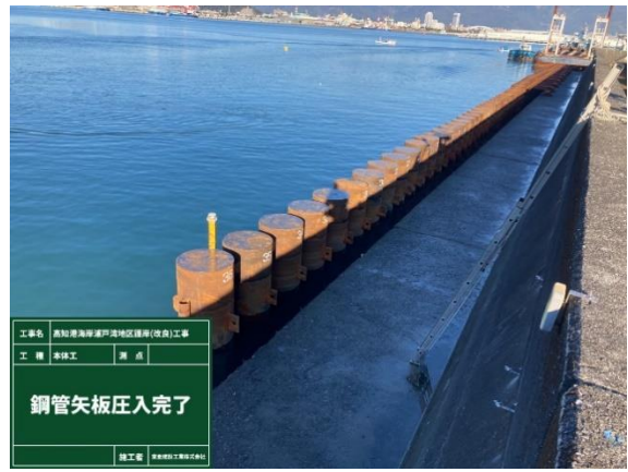
鋼管矢板打設完了状況
