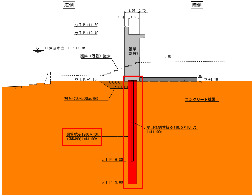
鋼管矢板打設作業
