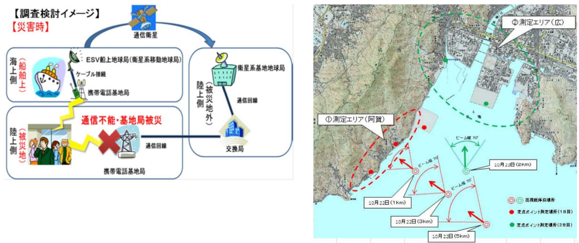
図 災害時における携帯電話基地局の船上開設に向けた検討イメージ
