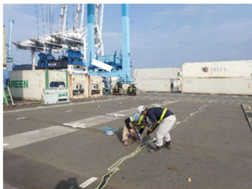
クラック等に充填剤を充填している様子（写真は他港の事例）
